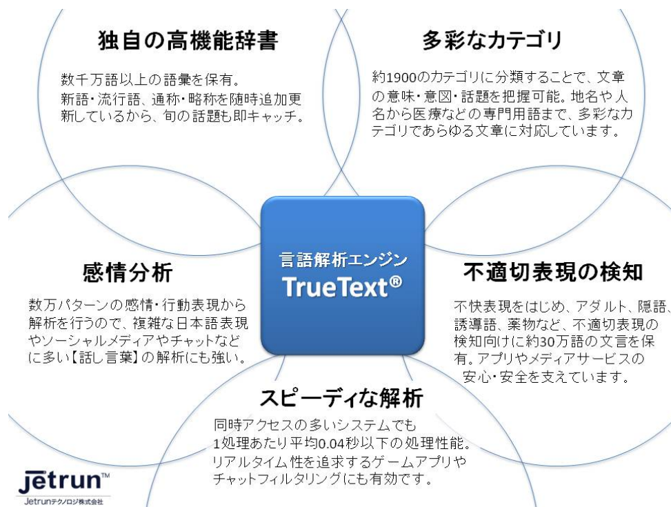
図 2.TrueText の概要
